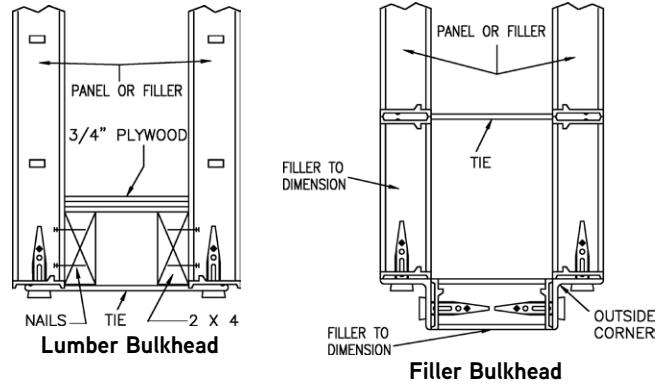
Filler Bulkhead
