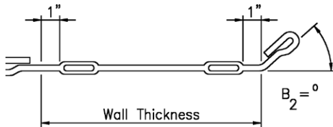
Pre-Bent Tie
